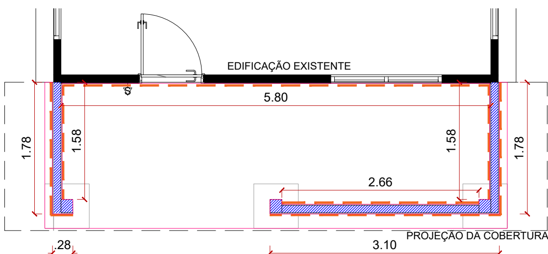
PROJETO PLANTA BAIXA REVESTIMENTO ESC: 1:50
