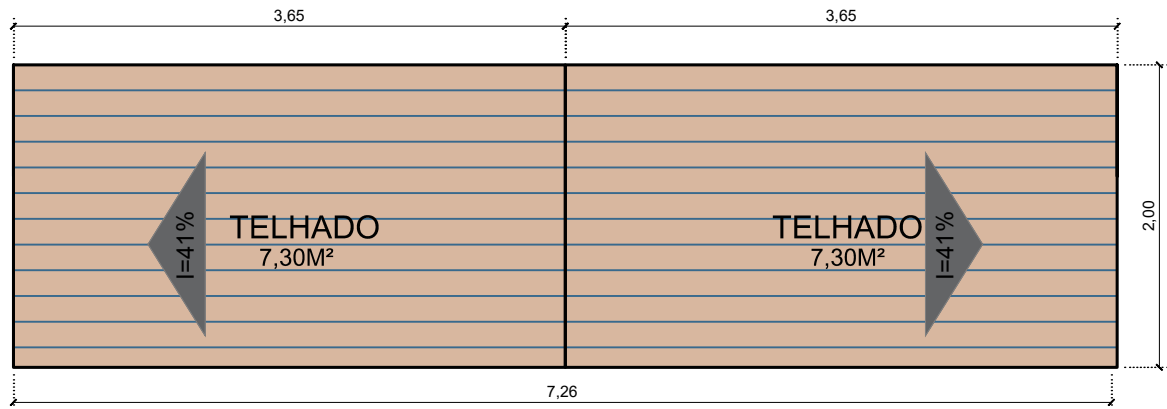
COBERTURA COBERTURA EM TELHA CERÂMICA ESC: 1:50
