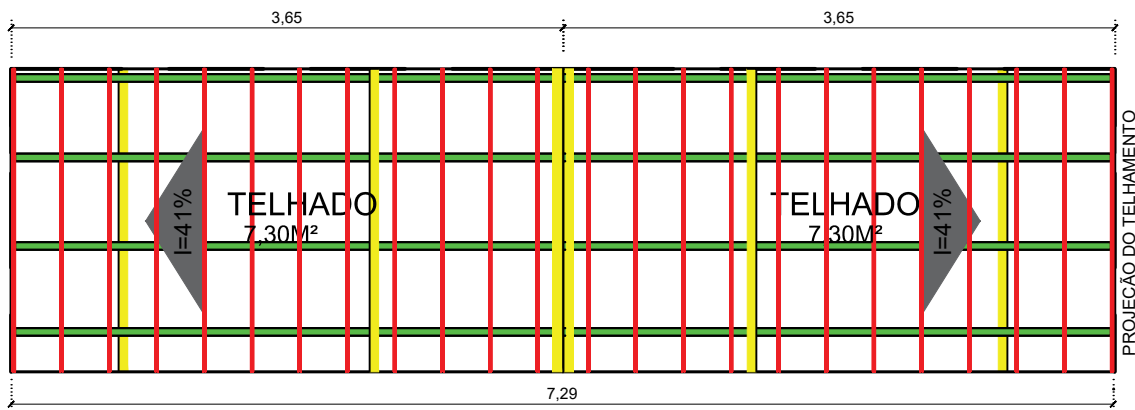
COBERTURA ESTRUTURA DA COBERTURA ESC: 1:50
