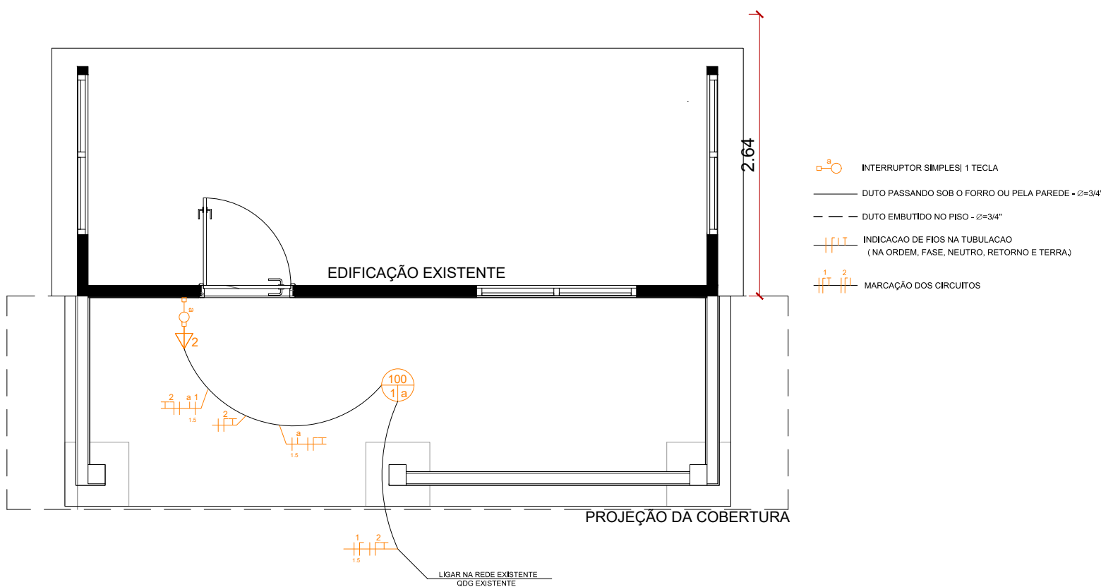
PROJETO PLANTA ELÉTRICA ESC: 1:50
